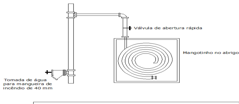
Figura 4: Sistema de mangotinho com válvula globo angular na prumada
