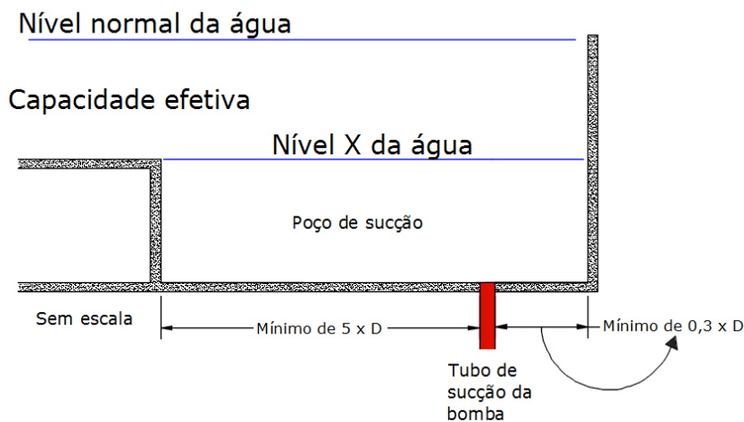
Figura 5 – Exemplo do item 6.2.3.2
