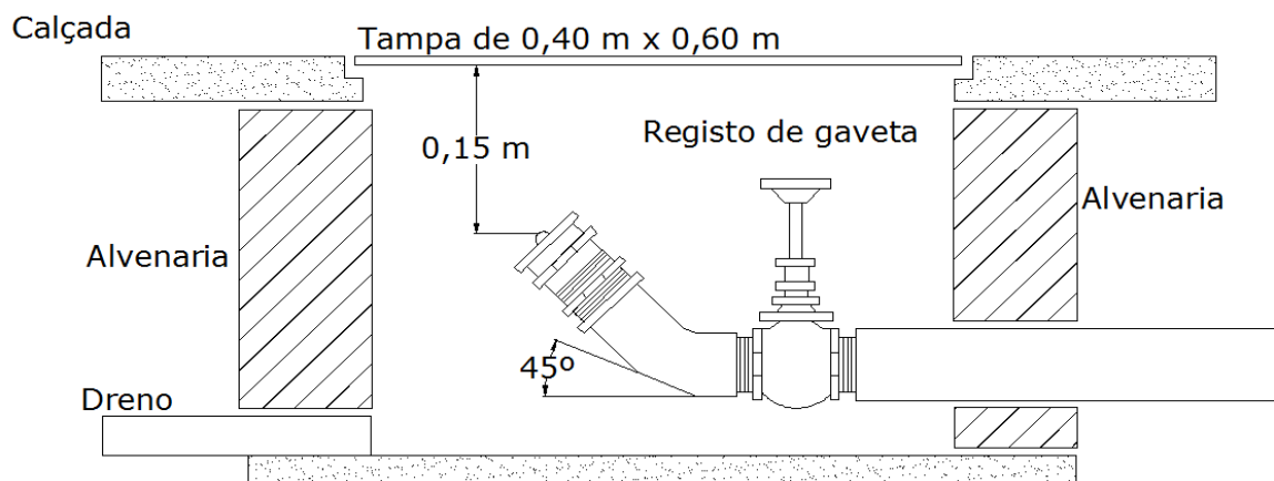
Figura 2 – Hidrante de recalque no passeio
