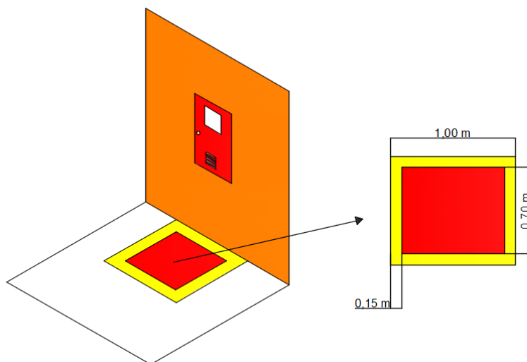
Figura 3: Sinalização de solo de acordo com o item 5.5.7
