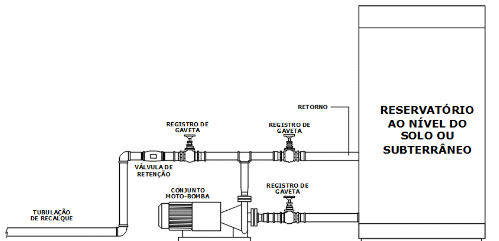
Figura 7 – Ilustrativa do item 6.2.3.5
